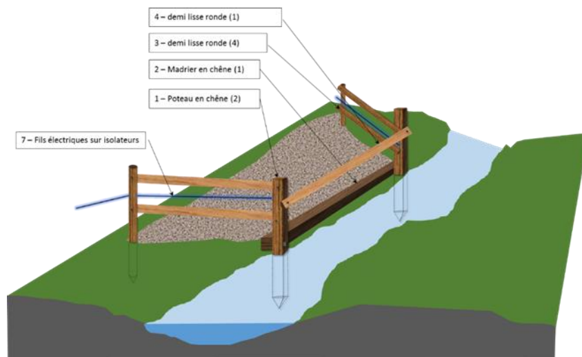
Figure 9 : Exemple d'abreuvoir stabilisé
