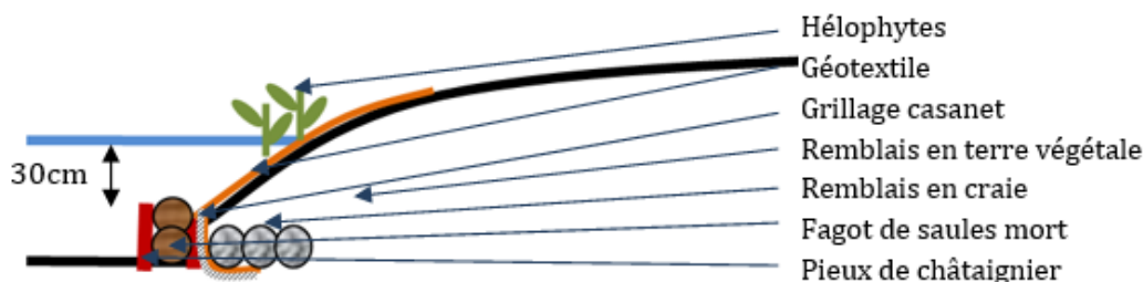
Figure 10 : Schéma de principe de fascinage d'hélophytes avec fascine de saule immergé
