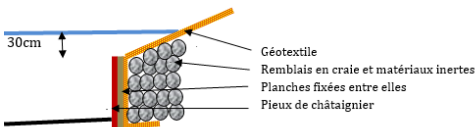
Figure 7 : Schéma de la technique de restauration de berge
