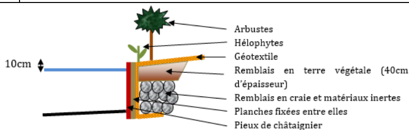
Figure 6 : Schéma de la technique de restauration de berge
